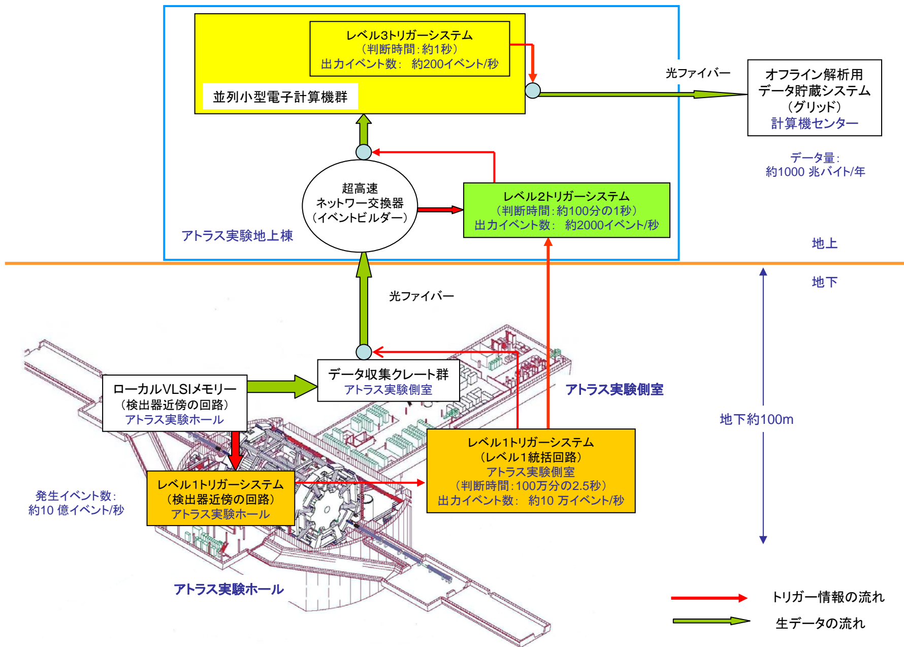
アトラス実験に使われるオンラインデータ収集法とトリガー
