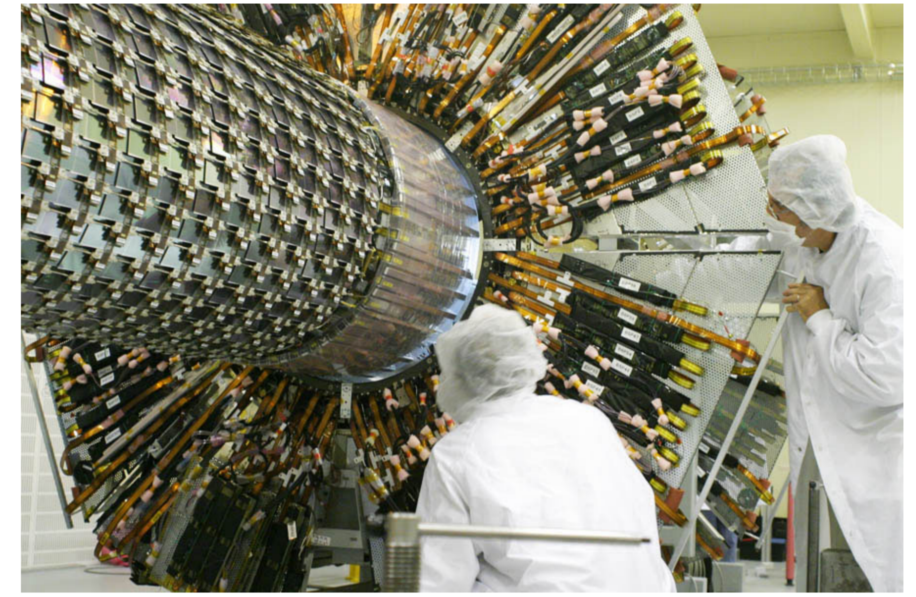
組立中のSCT(2005年9月@CERN)
