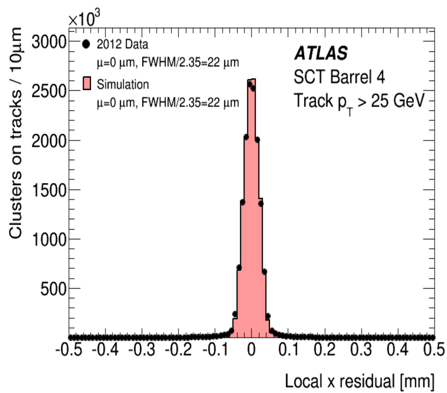
μ粒子飛跡とヒット位置の残差分布。(黒)データ(赤)MCシミュレーション
